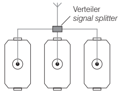
Sternanschaltung star connection
